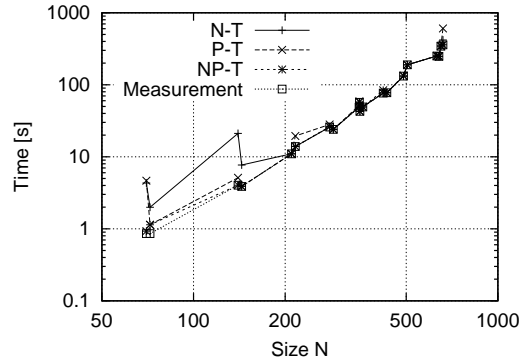
図 3 hpcmw-solver-test ( \log P の項を省いた場合)
