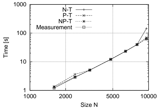
図 5 HPL
