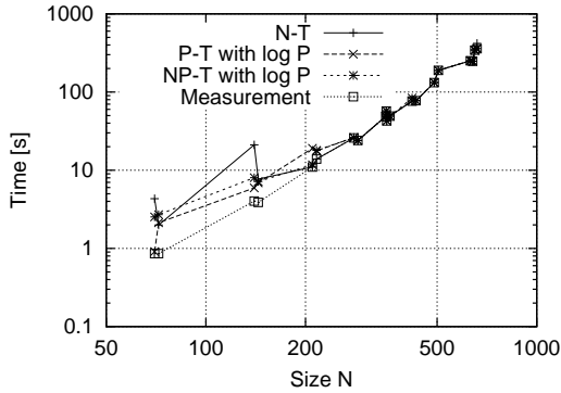
図 2 hpcmw-solver-test ( \log P の項がある場合)
