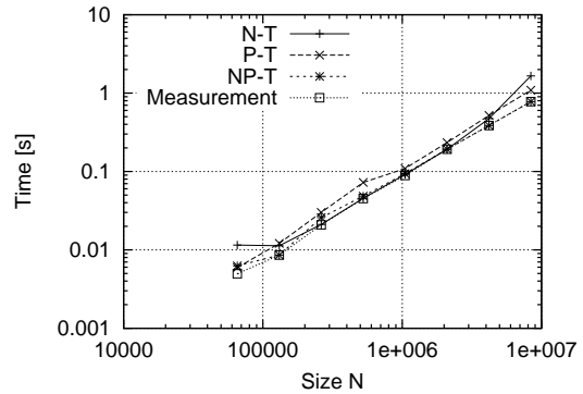
図 4 FFTE
