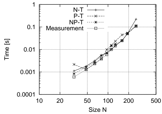
図 1 Himeno BMT
